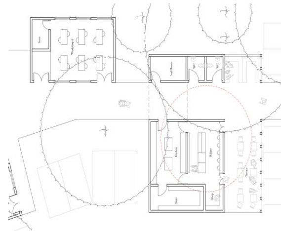
Erste Pläne der Bäckerei mit Café und Terrasse.
